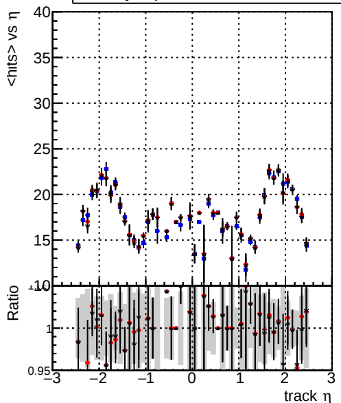
mean hits vs \eta DQMstep3_ZToEE_CKF DQMstep3_ZToEE_default DQMstep3_ZToEE_ckfPixelLess
