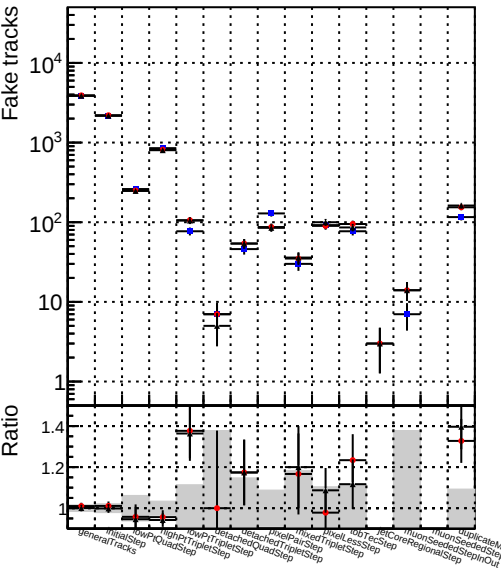
Number Variable 1 DQMstep3_ZToEE_default 2 DQMstep3_ZToEE_ckfPixelLess
