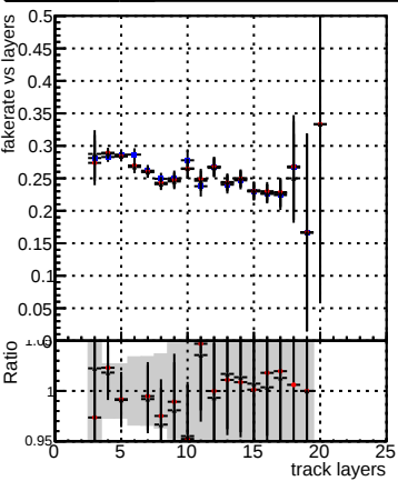
Legend: - DQMstep3_ZToEE_CKF (blue dots) - DQMstep3_ZToEE_default (red dots) - DQMstep3_ZToEE_ckfPixelLess (black dots)
