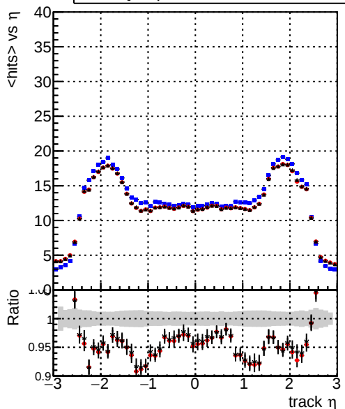
mean hits — DQMstep3_ZToEE_CKF — DQMstep3_ZToEE_default — DQMstep3_ZToEE_ckfPixelLess
