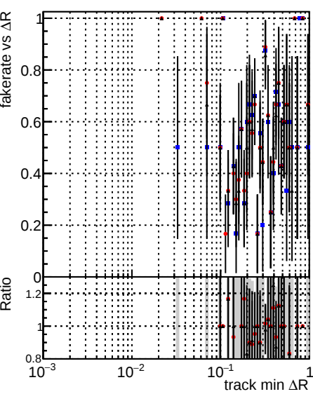
Fake rate vs \Delta R (track, jet) DQMstep3_ZToEE_CKF DQMstep3_ZToEE_default DQMstep3_ZToEE_ckfPixelLess
