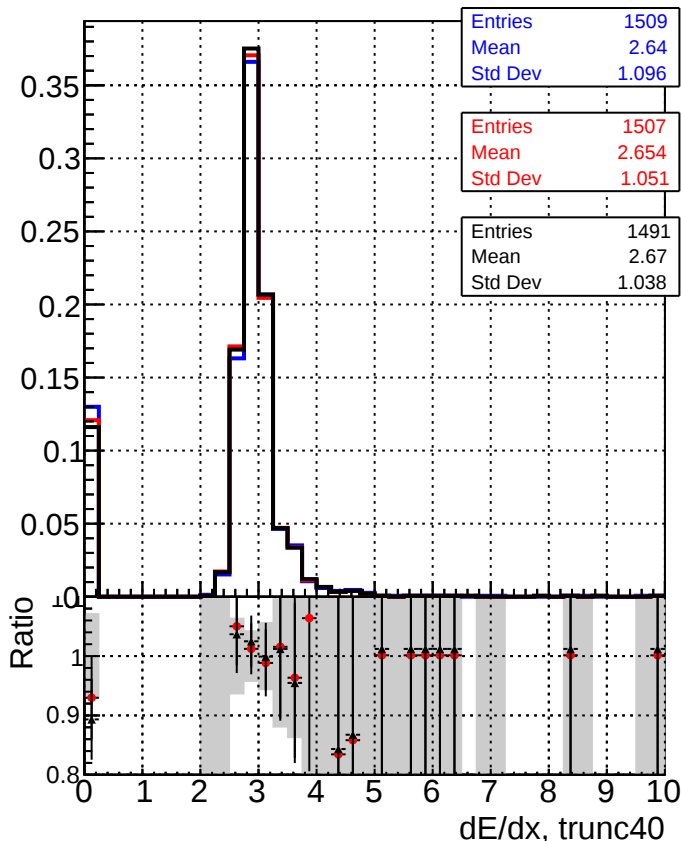
dE/dx estimator 2
