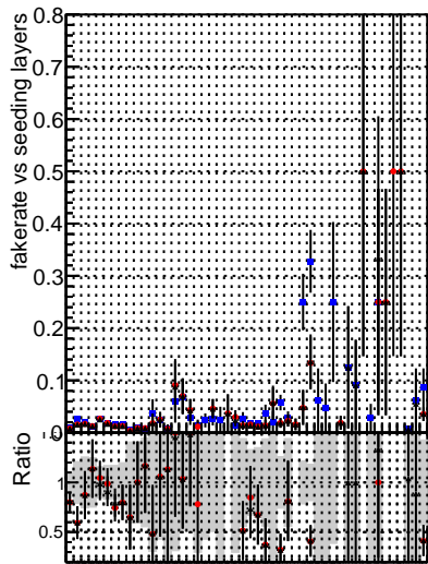
Fake rate vs. — DQMstep3 — ZToEE — GKF — default — CR — PixelLess
