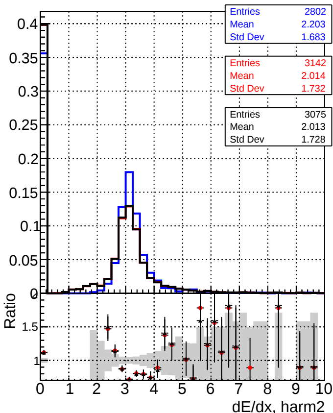
—■— DQMstep3_ZToEE_CKF —●— DQMstep3_ZToEE_default —■— DQMstep3_ZToEE_ckfPixelLess
