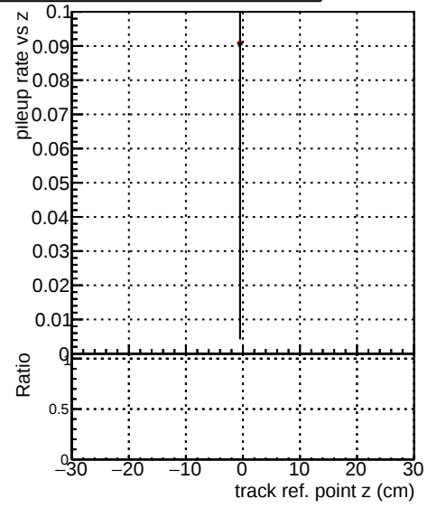
Legend: —•— DQMstep3_ZToEE_CKF —•— DQMstep3_ZToEE_default —•— DQMstep3_ZToEE_ckfPixelLess
