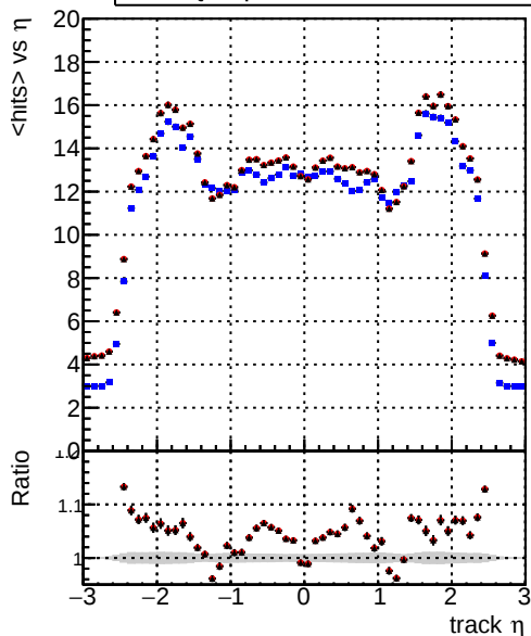
mean hits vs \eta — DQMstep3_ZToEE_CKF — DQMstep3_ZToEE_default — DQMstep3_ZToEE_ckfPixelLess
