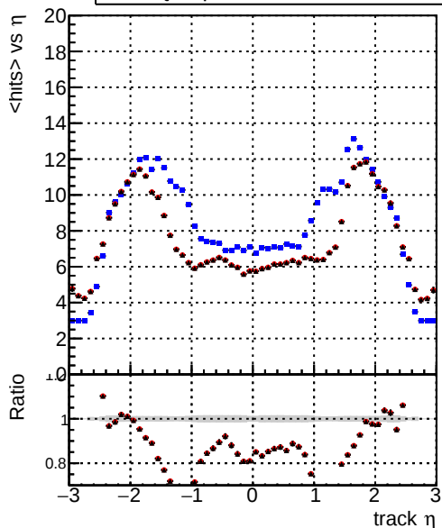
mean hits vs \eta — DQMstep3_ZToEE_CKF — DQMstep3_ZToEE_default — DQMstep3_ZToEE_ckfPixelLess
