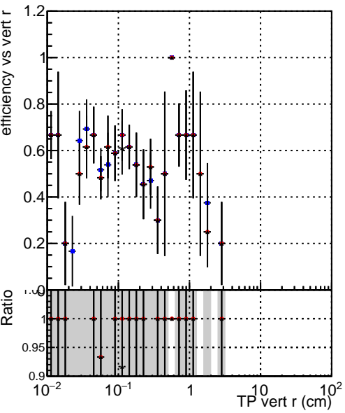
Efficiency vs vert r DQMstep3_ZToEE_CKF DQMstep3_ZToEE_default DQMstep3_ZToEE_ckfPixelLess
