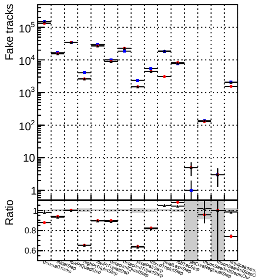
Number Variable 1 DQMstep3_ZToEE_default 2 DQMstep3_ZToEE_ckfPixelLess
