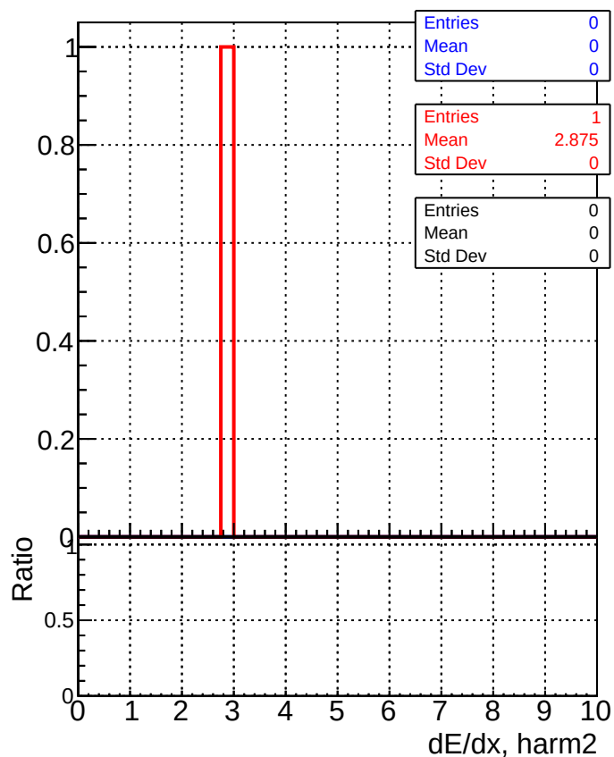
dE/dx estimator 1
