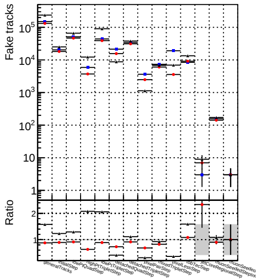
Number Parameter 1 DQMstep3_ZToEE_default 2 DQMstep3_ZToEE_defaultNEWT
