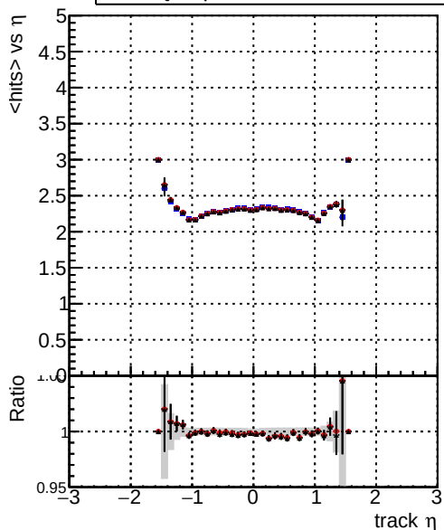
mean hits DQMstep3_ZToEE_CKF DQMstep3_ZToEE_default DQMstep3_ZToEE_defaultNEWT
