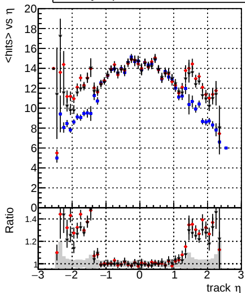
DQMstep3_ZToEE_CKF DQMstep3_ZToEE_default DQMstep3_ZToEE_defaultNEWT mean hits
