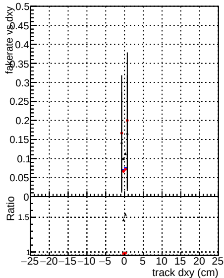
—•— DOMstep3 ZToEE CKF —•— DOMstep3 ZToEE default —•— DOMstep3 ZToEE NEWT
