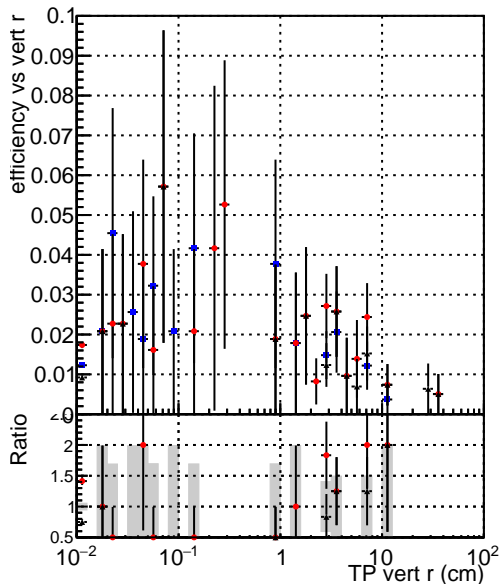
—●— DQMstep3_ZToEE_CKF —●— DQMstep3_ZToEE_default —●— DQMstep3_ZToEE_defaultNEWT
