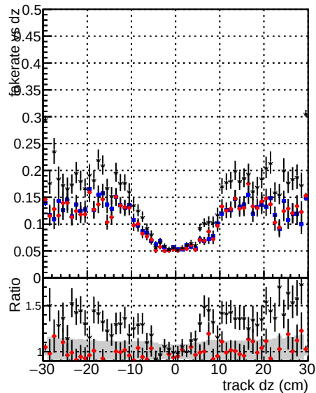
— DOMstep3 ZToFF CKF — DOMstep3 ZToFF default — DOMstep3 ZToFF default NEWT
