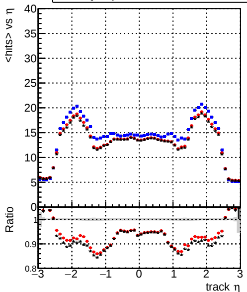
mean hits — DQMstep3_ZToEE_CKF — DQMstep3_ZToEE_default — DQMstep3_ZToEE_defaultNEWT
