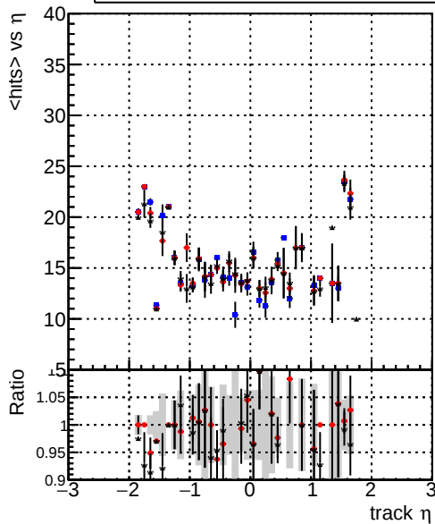
mean hit — DQMstep3_ZToEE_CKF — DQMstep3_ZToEE_default — DQMstep3_ZToEE_defaultNEWT
