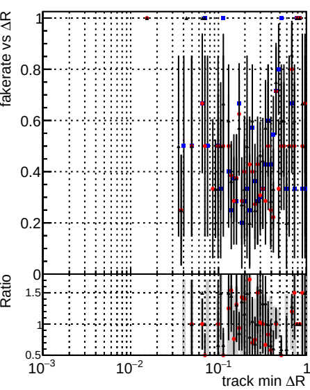
Fake rate vs \Delta R (track, jet) DQMstep3_ZToEE_CKF DQMstep3_ZToEE_default DQMstep3_ZToEE_defaultNEWT
