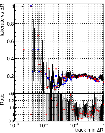
Fake rate vs \Delta R(\text{track, jet}) DQMstep3_ZToEE_CKF DQMstep3_ZToEE_default DQMstep3_ZToEE_defaultNEWT
