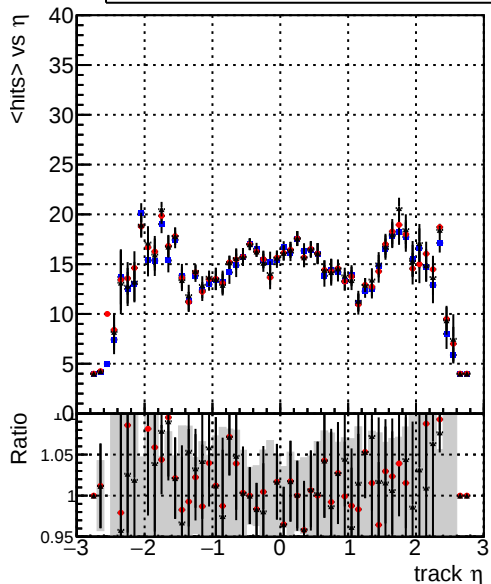
mean hit — DQMstep3_ZToEE_CKF — DQMstep3_ZToEE_default — DQMstep3_ZToEE_defaultNEWT
