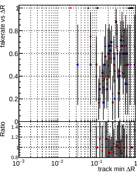
Fake rate vs ΔR(track, jet) DQMstep3_ZToEE_CKF DQMstep3_ZToEE_default DQMstep3_ZToEE_defaultNEWT
