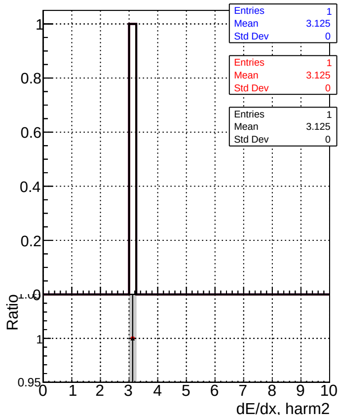
dE/dx estimator 1
