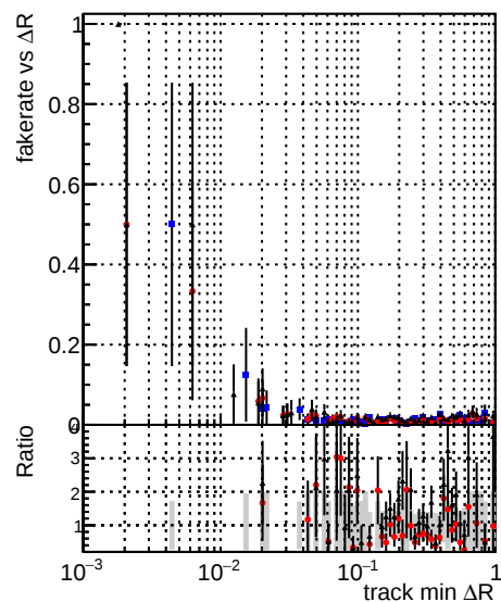
—●— DQMstep3_ZToEE_CKF —●— DQMstep3_ZToEE_default —●— DQMstep3_ZToEE_defaultNEWT
