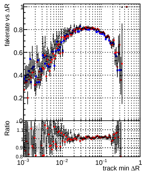
—●— DOMstep3_ZToEE_CKF —●— DOMstep3_ZToEE_default —●— DOMstep3_ZToEE_defaultNEWT
