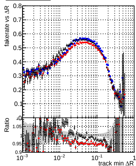
Legend: DQMstep3_ZToEE_CKF (black line) DQMstep3_ZToEE_default (red line) DQMstep3_ZToEE_defaultNEWT (blue line)
