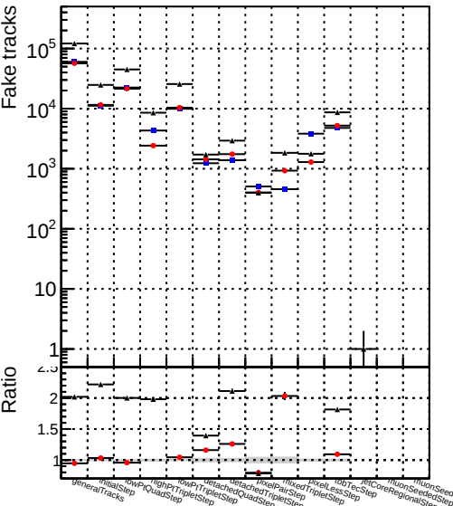
Number —●— DQMstep3_ZToEE_default —★— DQMstep3_ZToEE_defaultNEWT
