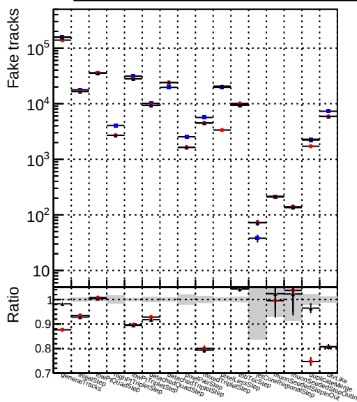
Number Legend 1 DQMstep3_TT_default 2 DQMstep3_TT_ckfPixelLess
