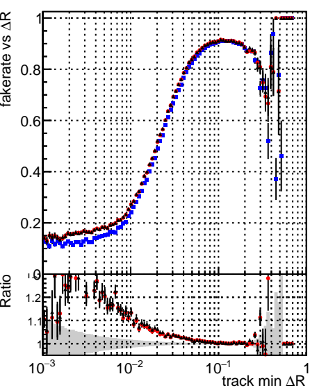
Fake rate vs \Delta R —●— DQMstep3_TT_CKF —●— DQMstep3_TT_default —●— DQMstep3_TT_ckfPixelLess
