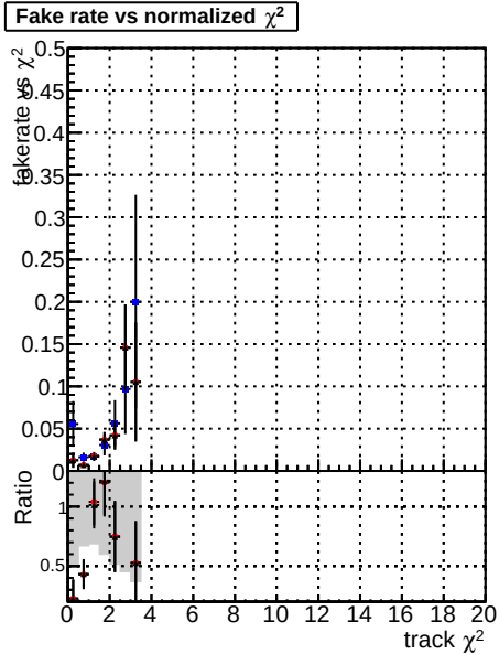
Fake rate vs. —•— DOMstep3 —•— CKF —•— default —+— DOMstep3 —+— CKF —+— PixelLess
