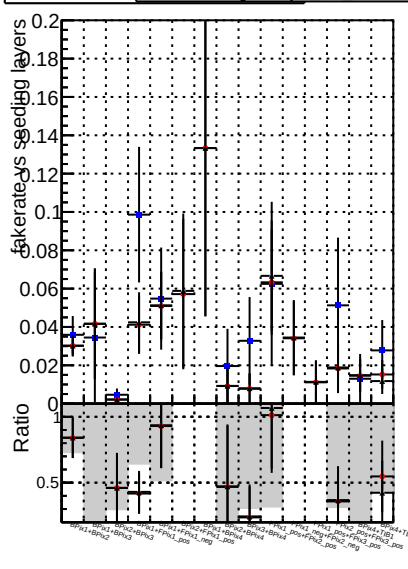
Fake rate vs. —•— DOMstep3 —•— CKF —•— default —+— DOMstep3 —+— CKF —+— PixelLess
