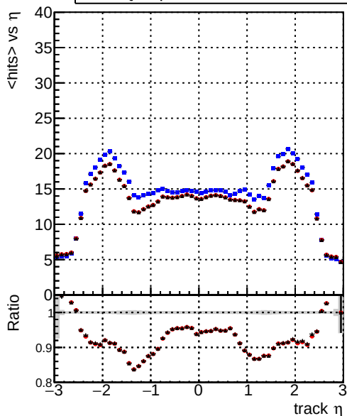
— DQMstep3_TT_CKF — DQMstep3_TT_default — DQMstep3_TT_ckfPixelLess mean hits
