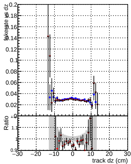
Fake rate vs dz —•— DOMstep3 TT CKF —•— DOMstep3 TT default —•— DOMstep3 TT CKFPixelLess
