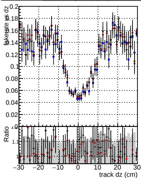
Fake rate vs d DOMstep3 CKF DOMstep3 default DOMstep3 CKFPixelLess
