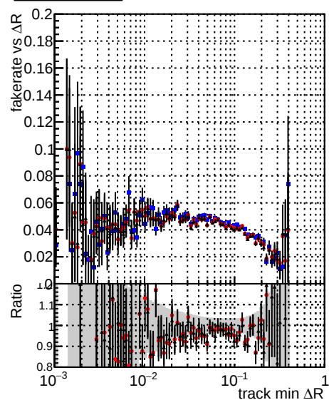
Legend: DQMstep3_TT_CKF (blue squares) DQMstep3_TT_default (red circles) DQMstep3_TT_ckfPixelLess (black crosses)
