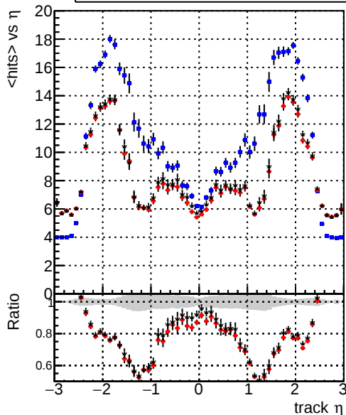
mean hit — DQMstep3_TT_CKF — DQMstep3_TT_default — DQMstep3_TT_ckfPixelLess
