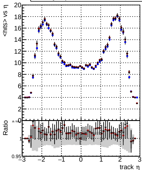
mean hits vs \eta — DQMstep3_TT_CKF — DQMstep3_TT_default — DQMstep3_TT_ckfPixelLess
