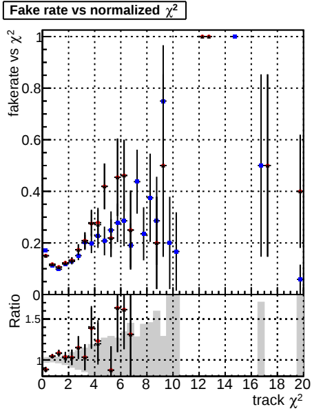
Fake rate vs. DOMstep3 CKF DOMstep3 default DOMstep3 CKFPixelLess
