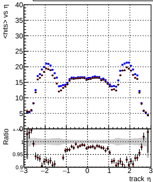
mean hit — DQMstep3_TT_CKF — DQMstep3_TT_default — DQMstep3_TT_ckfPixelLess
