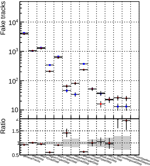
Number Legend ● DQMstep3_TT_default ▲ DQMstep3_TT_ckfPixelLess
