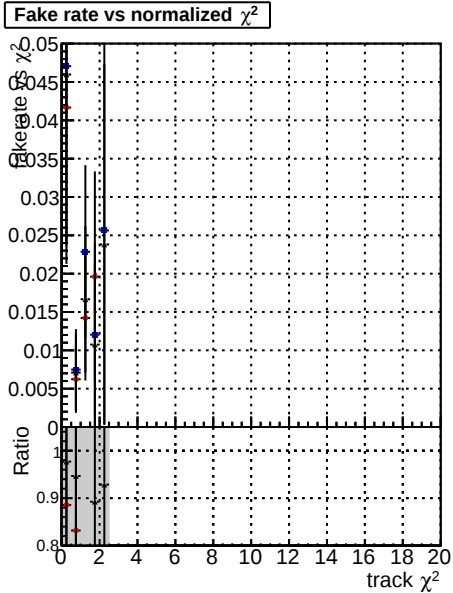
Fake rate vs. DOMstep3 TT CKF DOMstep3 default DOMstep3 CKFPixelLess
