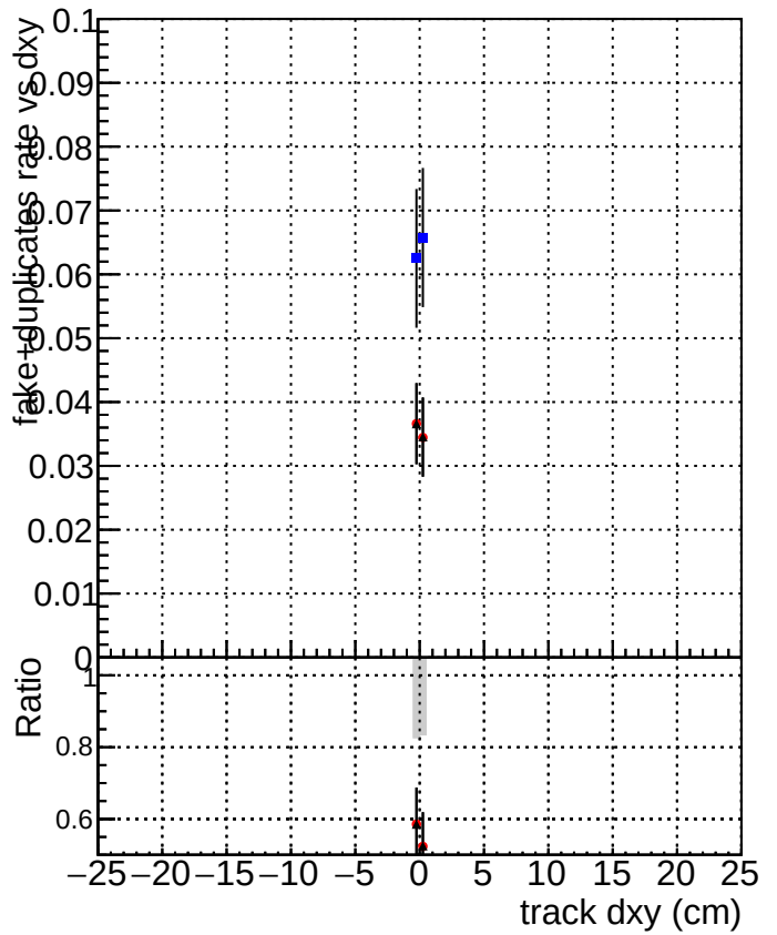
DQMstep3_TT_CKF DQMstep3_TT_default DQMstep3_TT_ckfPixelLess
