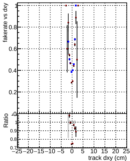
DOMstep3 TT CKF DOMstep3 default DOMstep3 ckfPixelLess
