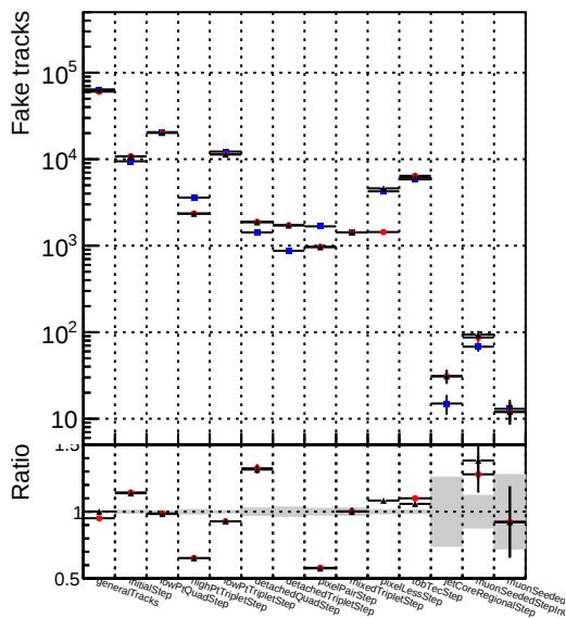
Number of tracks vs collection Legend: DQMstep3_TT_CKF DQMstep3_TT_default DQMstep3_TT_ckfPixelLess
