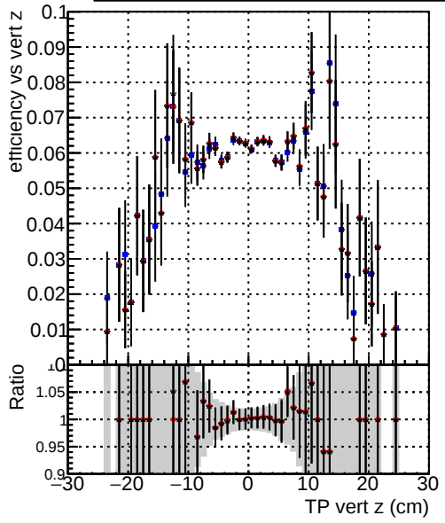
Efficiency vs. TP vert z (cm) —●— DQMstep3_TT_CKF —●— DQMstep3_TT_default —●— DQMstep3_TT_ckfPixelLess
