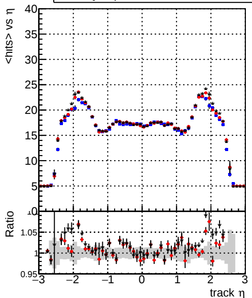
mean hits vs \eta — DQMstep3_TT_CKF — DQMstep3_TT_default — DQMstep3_TT_ckfPixelLess
