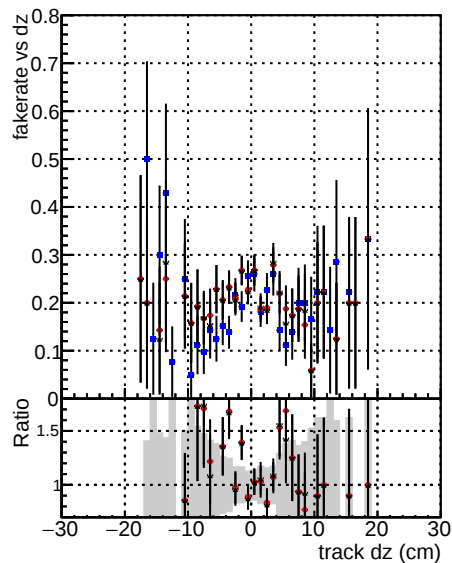
Fake rate vs dz DOMstep3 CKF DOMstep3 default DOMstep3 CKFPixelLess
